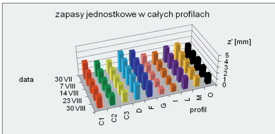
Rysunek 2. Zapasy jednostkowe wyliczone dla całej miąższości profili glebowych Figure 2. Unitary water storages calculated for the total depth of profiles
