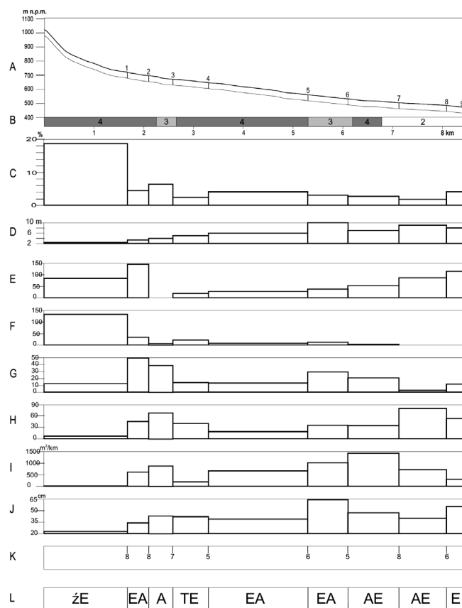
Rysunek 2. Struktura i typologia koryta potoku Hulskiego: A – profil podłużny koryta z granicami odcinków morfodynamicznych, B – uproszczona litologia (2 – łupki; 3 – łupki i piaskowce, 4 – piaskowce), C – spadek podłużny koryta w %, D – szerokość koryta w m, E – liczba progów skalnych na 1 km, F – liczba progów rumowiskowych na 1 km, G – liczba podcięć erozyjnych brzegu na 1 km, H – liczba łąch i wysp na 1 km, I – powierzchnia łąch w m 2 na 1 km, J – frakcja maksymalna rumowiska w cm,
