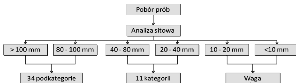
Rysunek 5. Schemat badań składu odpadów metodą SWA Tool Figure 5. Pattern of investigations of morphological composition municipal wastes by SWA Tool
