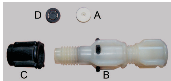
Rys. 1. Widok części rozpylacza sadowniczego z regulowaną wkładką wirową (fot. R. Skrzypniak): A - ceramiczny krążek wytryskowy KWP 010; B - króciec z regulowaną komorą wirową; C - nakrętka mocująca krążek (A); D - dwukanałowa wkładka wirowa z PCV
