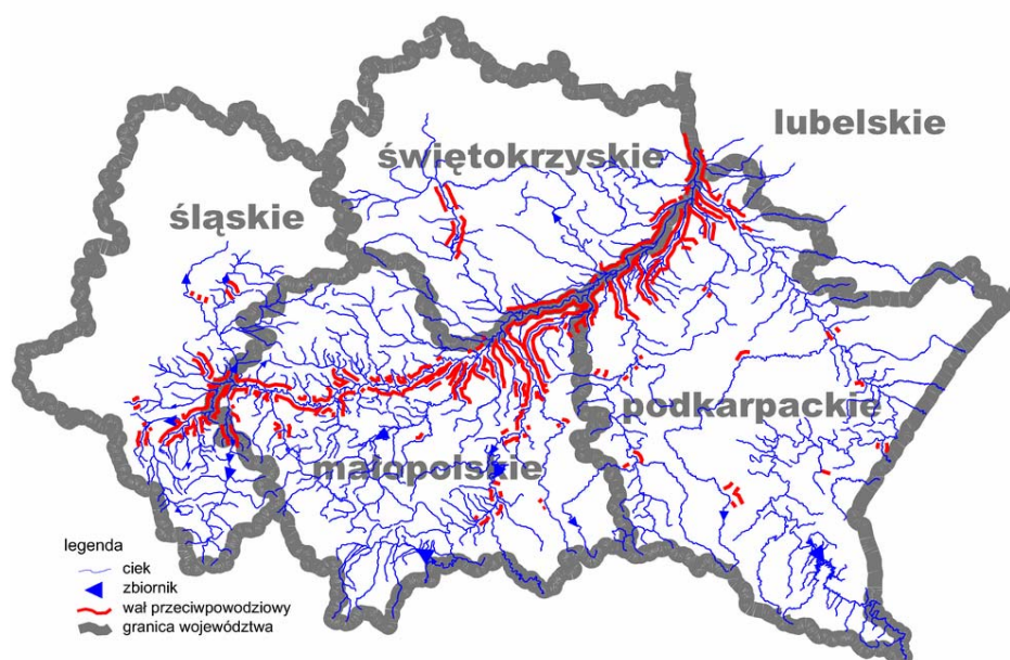
Rysunek 2. Podstawowe środki ochrony w Małopolsce i w dorzeczu górnej Wisły Figure 2. Basic flood control measures in Małopolska and upper Vistula region
