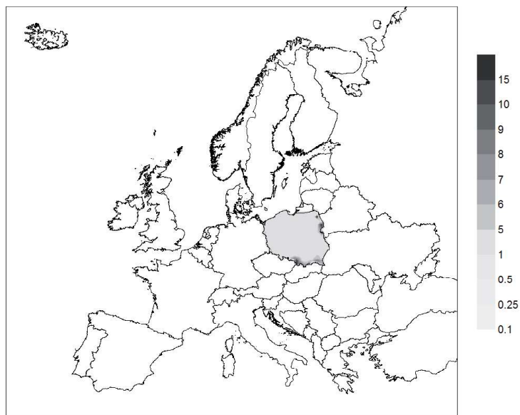
RYSUNEK 3. Depozycja kadmu [ \text{mg}/\text{m}^2 ] w 2012 roku na obszarze Polski w wyniku emisji ze wszystkich źródeł w domenie obliczeniowej z wyjątkiem zlokalizowanych w Polsce (zob. objaśnienia w tekście; punkt 2 – „import” zanieczyszczeń)
