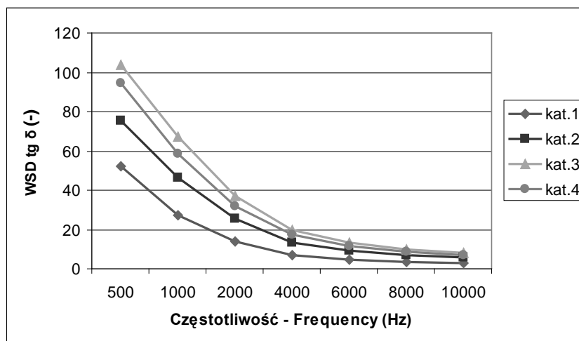
Rys. 1. Zależność między częstotliwością (500-10000 Hz) a wartością współczynnika strat dielektrycznych (WSD) \text{tg } \delta dla różnych kategorii miodów (1-4)
