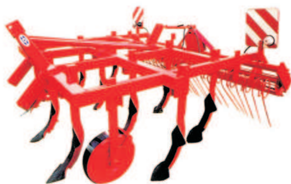
Rys. 1. Kultywator podorywkowy U 427, prod. Agromet Jawor Zakład Mechaniczny Sp. z o.o.; [www.agromet-jawor.pl]
