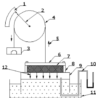
Rys. 2. Schemat przyrządu do oznaczania przepuszczalności powietrznej gleby: 1 - skala pomiarowa, 2 - wskazówka, 3 - szalka z obciążnikiem, 4 - obrotowa tarcza, 5 - kierunek ruchu pływaka, 6 - strzemię dociskające cylinderek wypełniony glebą do pływaka, 7 - badana próbka gleby, 8 - cylinderek, 9 - pływak, 10 - przewód zakończony U-rurką, 11 - zbiornik napełniony wodą, 12 - kierunek przepływu powietrza
