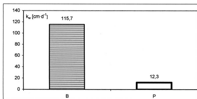
Rys. 4. Wartości współczynnika filtracji podornej warstwy gleby po uprawie płuznej (P) oraz po uprawie bezorkowej (B) Fig. 4. Values of filtration coefficient of the subsoil layer after plough tillage (P) as well as after no tillage (B)
