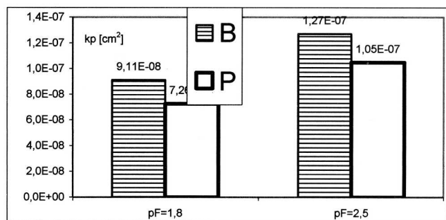
Rys. 5. Przepuszczalność powietrzna ( k_p ) podornej warstwy gleby po uprawie płuznej (P) oraz po uprawie bezorkowej (B) Fig. 5. Air penetrability ( k_p ) of subsoil layer after plough tillage (P) as well as after no tillage (B)
