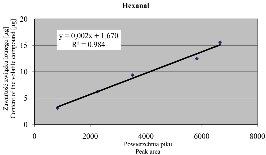
Rys. 7. Krzywa wzorcowa hexanal.
