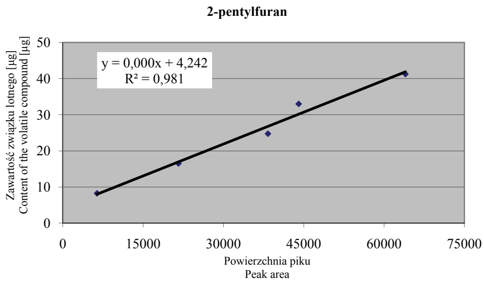
Rys. 8. Krzywa wzorcowa 2-pentylfuranu.
