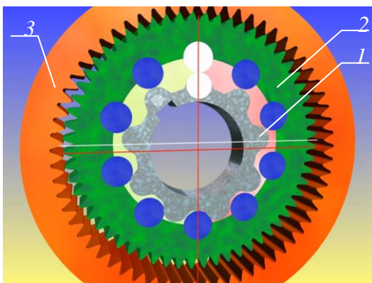
Рис. 3. Схема движения вытеснителей в планетарных гидромоторах семейства унифицированных рядов ПРГ-33, ПРГ-22, ПРГ-11, и ПРГ-8: 1 – охватываемый вытеснитель (солнечная шестерня); 2 – охватывающий вытеснитель (сателлит); 3 – корпус (коронная шестерня)
