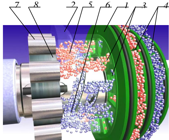
Рис. 4. Принцип работы торцевого распределения рабочей жидкости: 1 – золотник; 2 – распределитель; 3 – распределительные окна; 4 – кольцевые каналы; 5 – зона нагнетания; 6 – зона слива; 7 – охватывающий вытеснитель; 8 – охватываемый вытеснитель
