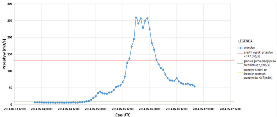
Rysunek 2. Hydrogram przepływu rzeki Kamienica Nawojowska ( www.pogodynka.pl )
