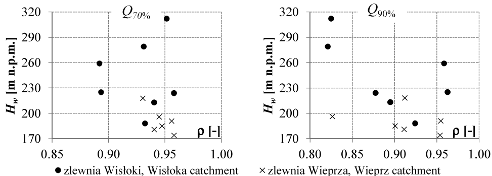
RYSUNEK 8. Współczynnik korelacji liniowej Pearsona ( \rho ) czasu trwania niżówki i jej deficytu zestawiony od wysokości położenia zera wodowskazu ( H_w ) w zlewniach Wisłoki i Wieprza dla Q_{70\%} i Q_{90\%}
