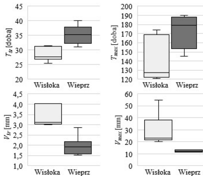
RYSUNEK 5. Średnie ( T_{sr} ) i maksymalne ( T_{max} ) czasy trwania niszówki oraz średnie ( V_{sr} ) i maksymalne ( V_{max} ) objętości niszówki w zlewniach Wisłoki i Wieprza przy Q_{70\%} FIGURE 5. Mean ( T_{sr} ) and maximal ( T_{max} ) low flow duration time and mean ( V_{sr} ) and maximal ( V_{max} ) flow deficit in Wisłoka and Wieprz catchments at Q_{70\%}
