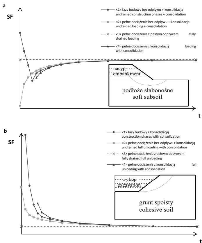
Rys. 3. Zmiana współczynnika stateczności w czasie w zależności od przyjętych warunków odpływu i obciążenia (objaśnienia w tekście): a – nasyp na słabym podłożu, b – wykop w gruntach spoiwych
