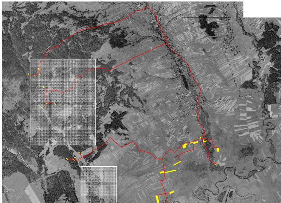
Rysunek 4. Gospodarstwo 262 (stan po scaleniu). Rozmieszczenie działek wchodzących w skład gospodarstwa wraz z najkrótszą siecią dróg łączących siedlisko gospodarstwa z działkami
