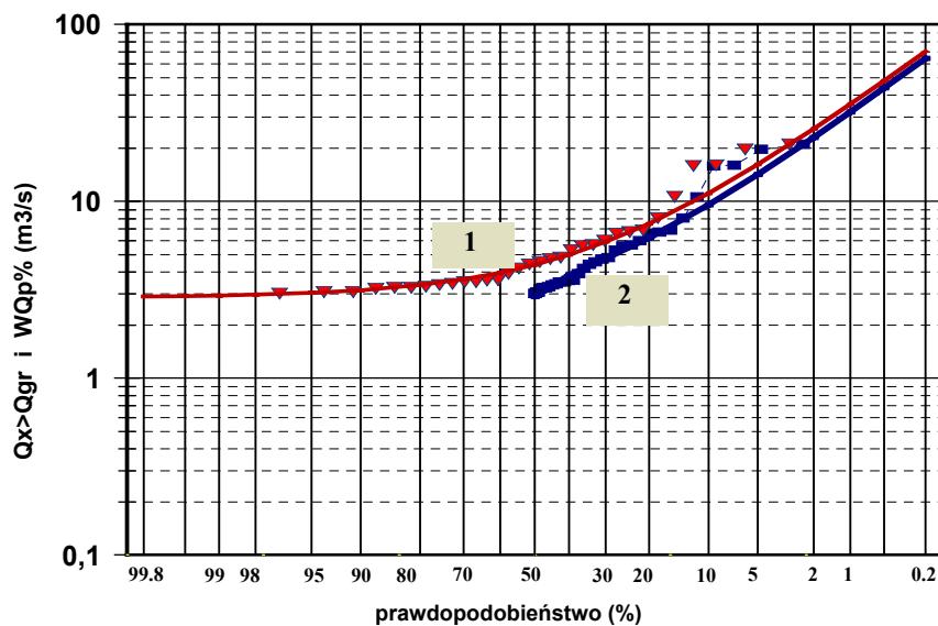
Rysunek 4. Krzywe prawdopodobieństwa zbioru POT przepływów maksymalnych Q_{\max} > Q_{\text{gr}} : 1 – dla prawdopodobieństwa w zbiorze, 2 – dla prawdopodobieństwa w roku
