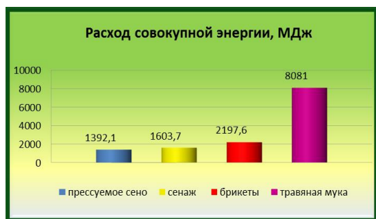
Рис. 3. Расход совокупной энергии на приготовление кормов из 1000 т зеленой массы
