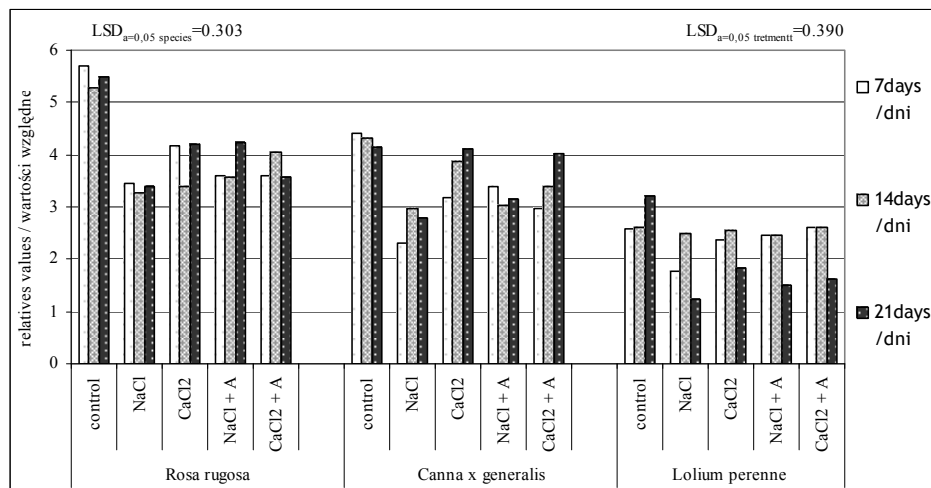
Fig. 8. Performance Index for Canna × generalis , Rosa rugosa L., Lolium perenne L. treated with road de-icing substances of 15, 5 and 10 g·dm -3 respectively, A: additives Ryc. 8. Wskaźnik funkcjonowania PS II roślin Canna × generalis , Rosa rugosa L., Lolium perenne L. traktowanych preparatami do odładzania ulic w ilości odpowiednio 15, 5 lub 10 g·dm -3 , A: dodatki
