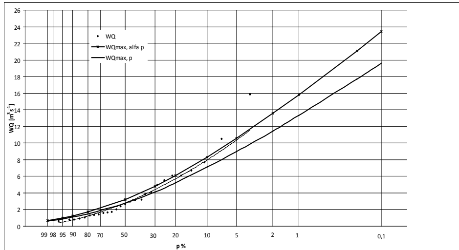
Rysunek 3. Krzywa prawdopodobieństwa przewyższenia maksymalnych przepływów rzeki Małej Wełny w przekroju Kiszkowo
