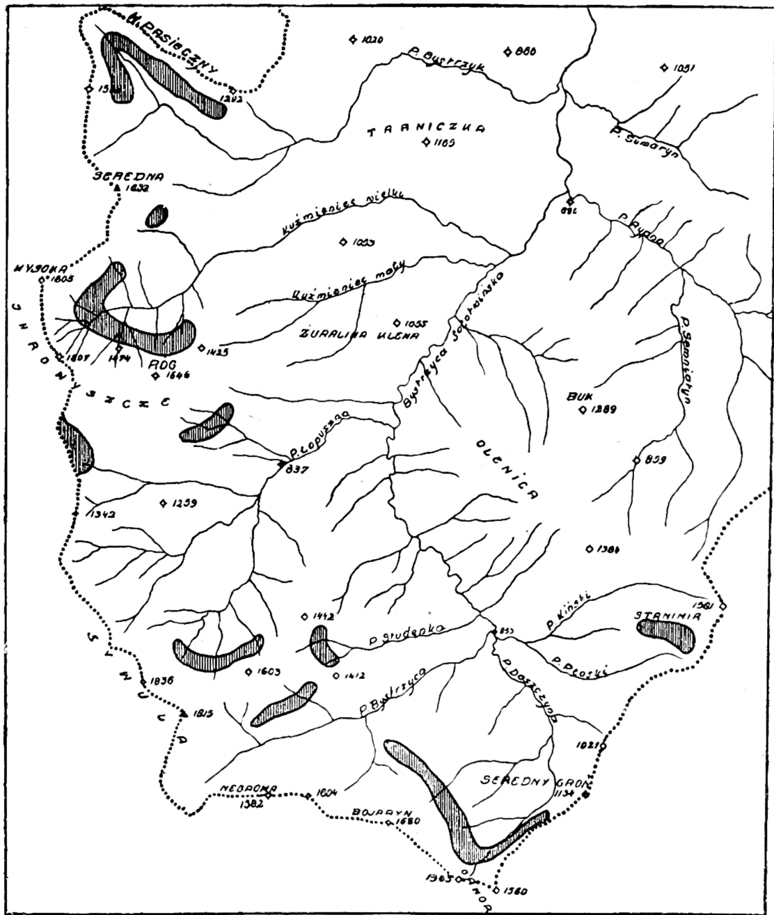
Ryc. 2. Rozmieszczenie limby u źródeł Bystrzycy Sołotwińskiej. (Pola zakreskowane oznaczają stanowiska z limbą).
