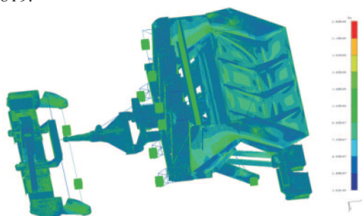
Rys. 8. Naprężenia zredukowane von Misesa [Pa], przypadek LC1, widok z góry
