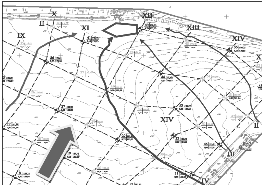
Rys. 2. Lokalizacja zbiornika, geotechnicznych punktów badawczych i zasadnicze kierunki splywu powierzchniowego Fig. 2. Location of reservoir and geotechnical research points, the main lines of surface runoff
