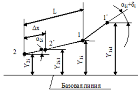
Рис. 2. Схема движения колесной машины вдоль базовой линии: L – длина колесной базы трактора; \alpha_1 – угол поворота передних управляющих колес; \alpha_2 – текущее значение курсового угла остова трактора; Y_1, Y_2 – текущее значение отклонений от базовой линии переднего и заднего колес трактора соответственно; \Delta X – шаг квантования модели по перемещению
