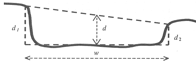
Rys. 1. Przekrój poprzeczny żłobin użyty do obliczeń
