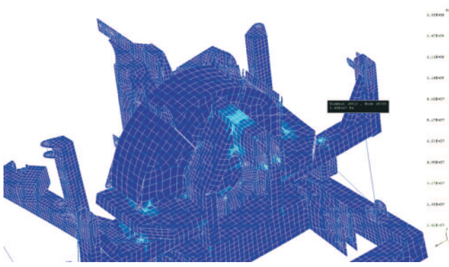
Rys. 3. Maszyna do zbioru wierzby krzewiastej metodą jednoetapową - naprężenia zredukowane Misses'a - widok ramy nošnej - przypadek transportu
