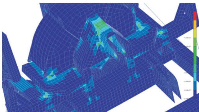
Rys. 2. Maszyna do zbioru wierzby krzewiastej metodą jednoetapową - naprężenia zredukowane Misses'a - widok ramy nošnej - przypadek hamowania
