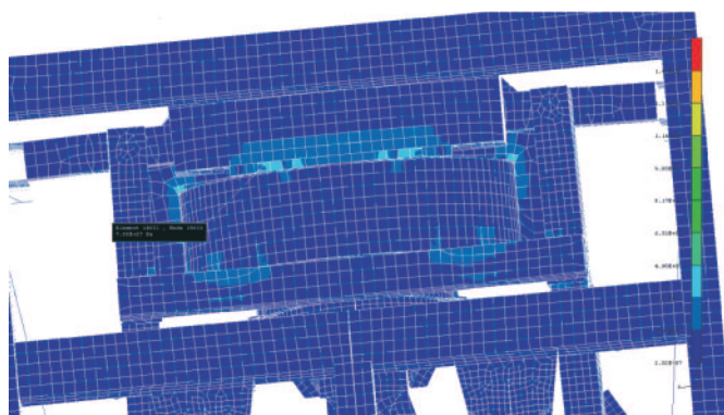
Rys. 3. Maszyna do zbioru wierzby krzewiastej metodą jednoetapową - naprężenia zredukowane Misses'a - widok ramy nošnej - przypadek transportu
