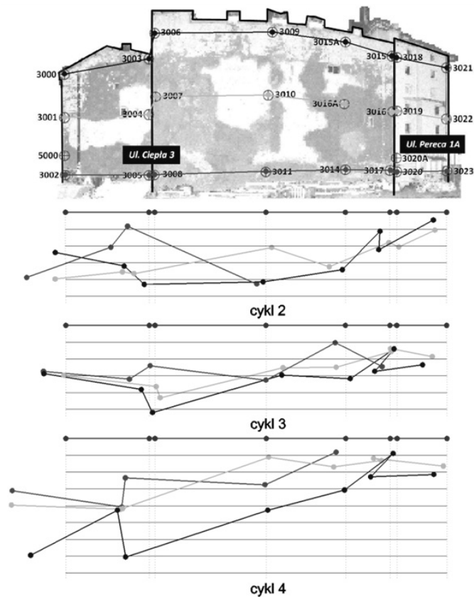
Rys. 3. Lokalizacja i wykresy względnych przemieszczeń punktów kontrolowanych na ścianach północnych budynków Ciepła 3 i Pereca 1A. Interwał linii poziomych na wykresie – 1,0 mm [Popielski i in. 2012]
