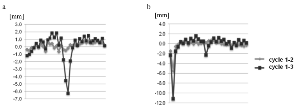
Rys. 7. Przemieszczenia punktów kontrolowanych profili: a – profil zachodni (od strony Ronda ONZ), b – profil wschodni (od strony Ronda Daszyńskiego)
