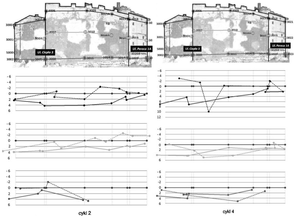
Rys. 5. Porównanie przemieszczeń poziomych punktów kontrolowanych na ścianach północnych budynków Ciepla 3 i Pereca 1A uzyskanych metodami klasycznymi (linia ciągła) i za pomocą skaningu laserowego (linia przerywana) Fig. 5. Comparison of vertical displacements of controlled points on the northern walls Ciepla 3 and Pereca 1A buildings obtained by classical methods (straight line) and with aid of the laser scanning (drop line)
