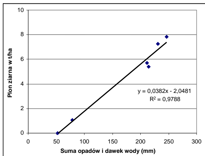
Rysunek 1. Zależność plonów ziarna od sumy opadów atmosferycznych i dawek nawadnieniowych w okresie czerwca i lipca Figure 1. Grain yields of maize as dependent on total rainfall and irrigation doses in June and July
