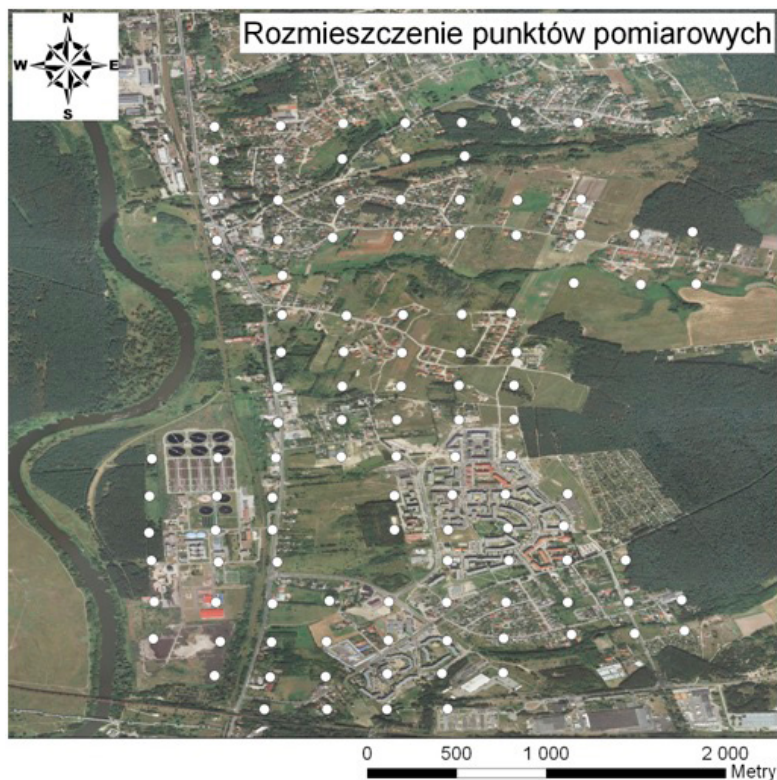
Rysunek 1. Siatka pomiarowa wyznaczona dla terenowych pomiarów imisji zapachu i oceny uciążliwości
