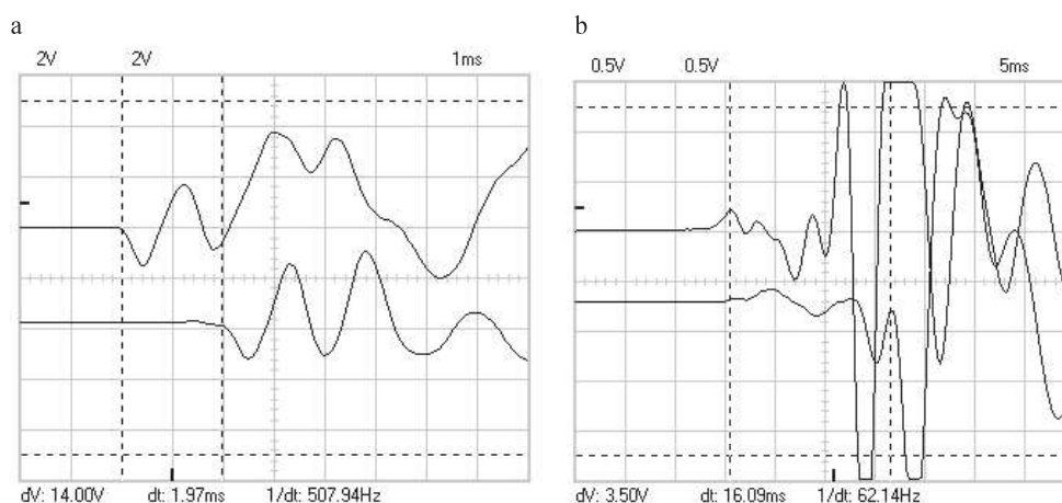
RYSUNEK 1. Przykładowe wyniki badań terenowych sondą SCPTU (metoda odczytu czasu propagacji fali poprzecznej: a – first deflection, b – peak-to-peak) FIGURE 1. The example of SCPTU test results (the travel time estimation by: a – first deflection, b – peak-to-peak method)
