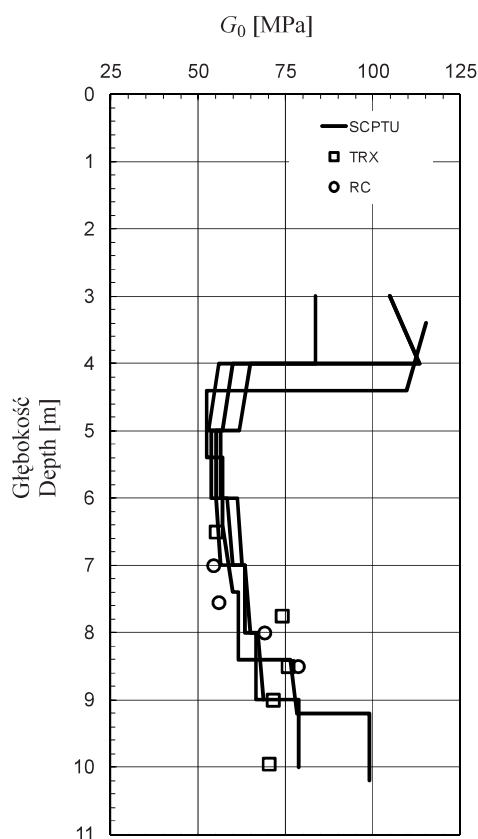
RYSUNEK 6. Początkowy moduł odkształcenia postaciowego otrzymany z badań terenowych (SCPTU) i laboratoryjnych (TRX i RC)
