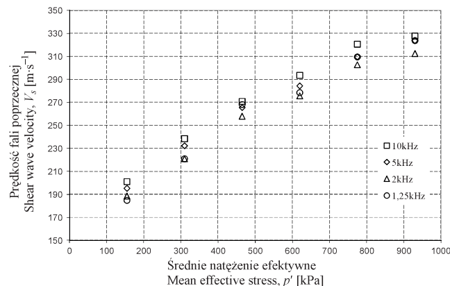
RYSUNEK 3. Przykład zależności między prędkością fali poprzecznej i napięciem efektywnym przy różnej częstotliwości nadawanego sygnału dla próbki pobranej z głębokości 7,75 m – metoda peak-to-peak (Markowska-Lech i in., 2015)
