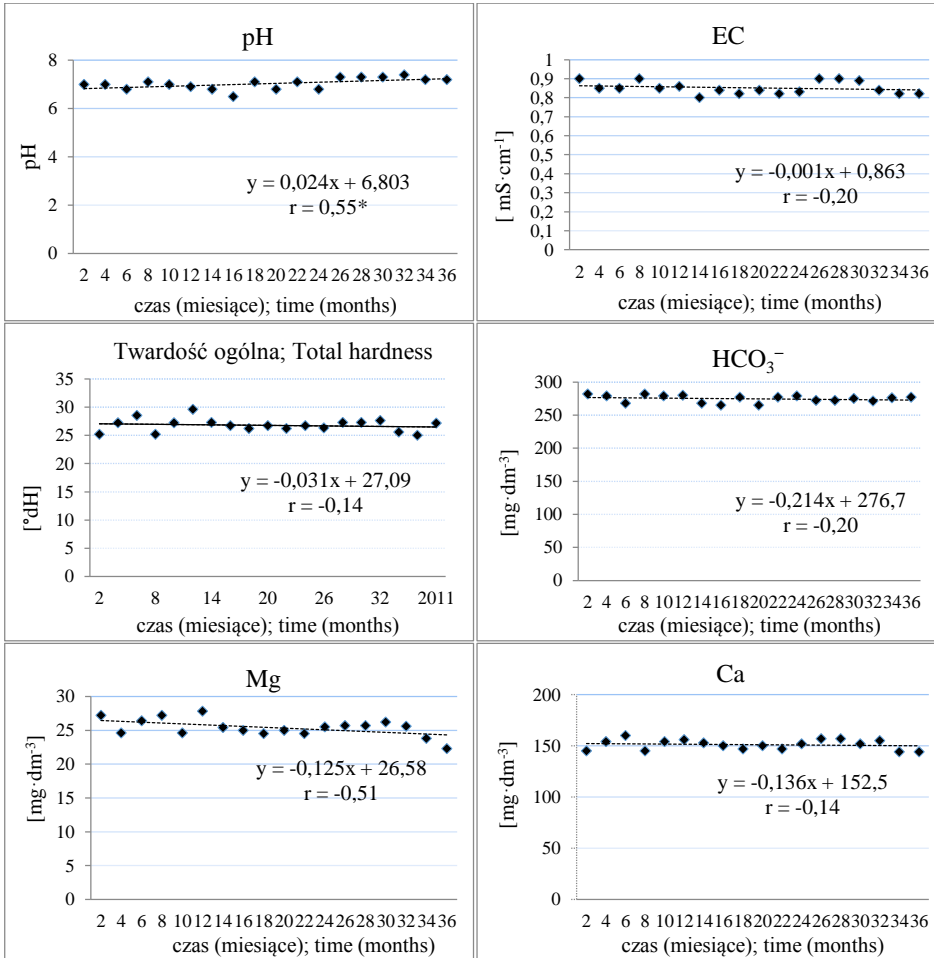
Rys. 4. Przebieg zmian właściwości fizyko-chemicznych wody w ujęciu zlokalizowanym w miejscowości Bukówiec Górny gm. Włoszakowice, pow. leszczyński w latach 2011-2013 (* – istotne przy p = 0,05 ; ** – istotne przy p = 0,01 )
