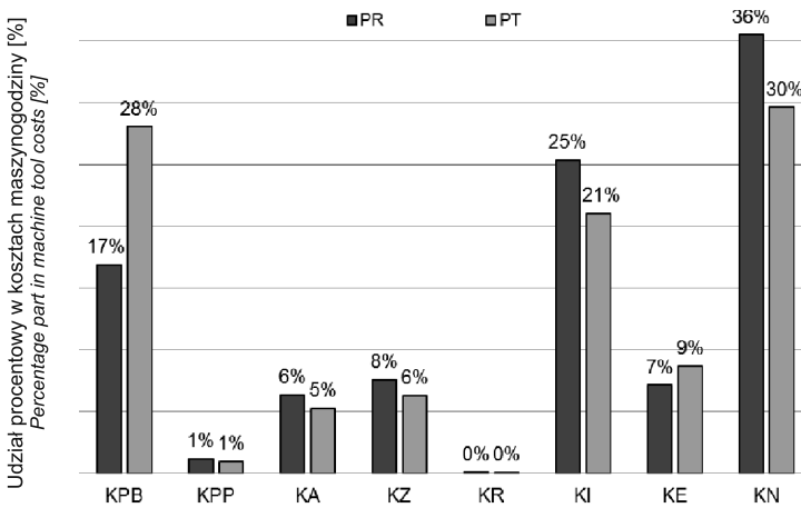
Rys. 4. Struktura kosztów maszynogodziny pilarki ramowej wielopilowej i pilarki taśmowej wraz z udziałem kosztów narzędziowych podczas produkcji deszczulek warstw licowych podłóg klejonych warstwowo (oznaczenia takie same jak w zależności (3))
