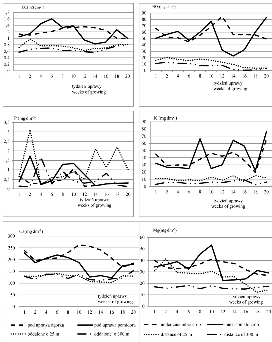
Rysunek 1. Wpływ bezglebowych upraw szklarniowych na zmiany EC, N-NO 3 , P, K, Ca i Mg w wodach gruntowych
