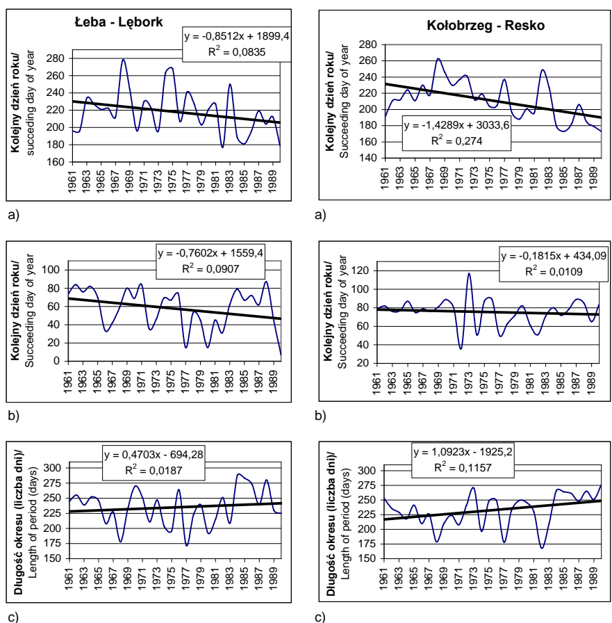
Rys. 2. Zmienność a) początku i b) końca oraz c) długości okresu z ocieplającym wpływem Bałtyku na termikę powietrza w strefie wybrzeża wraz z trendami w latach 1961-1990 na przykładzie relacji między temperaturami w Łebie i Lęborku oraz Kołobrzegu i Resku
