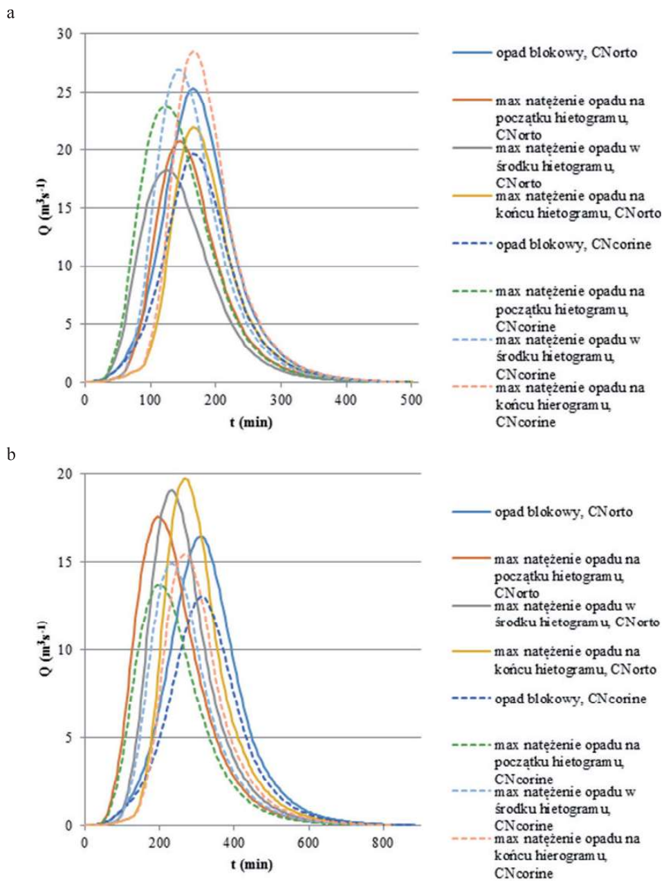
RYSUNEK 2. Hydrogram odpływu bezpośredniego dla zlewni rzeki Sidzinki: (a) T_{cTR-55} , (b) T_{cKerby-Kirpich} (opracowanie własne)
